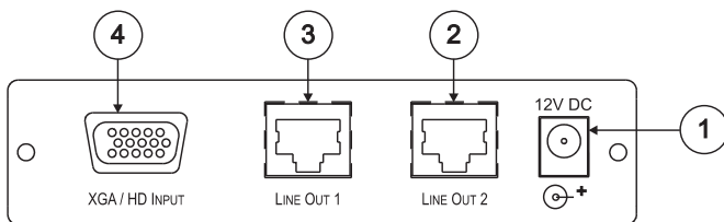
Рис. 2. TP-112HD (разъемы на верхней панели)
