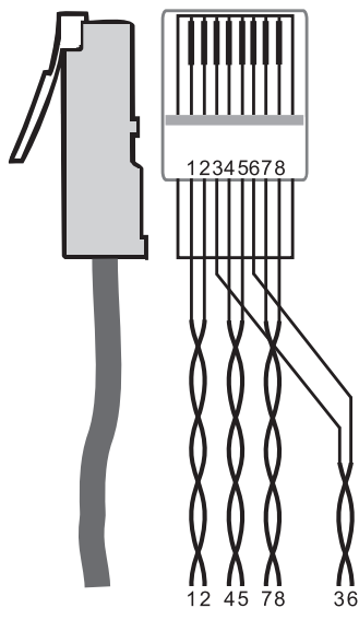
Рис. 6. Разводка соединительного кабеля
