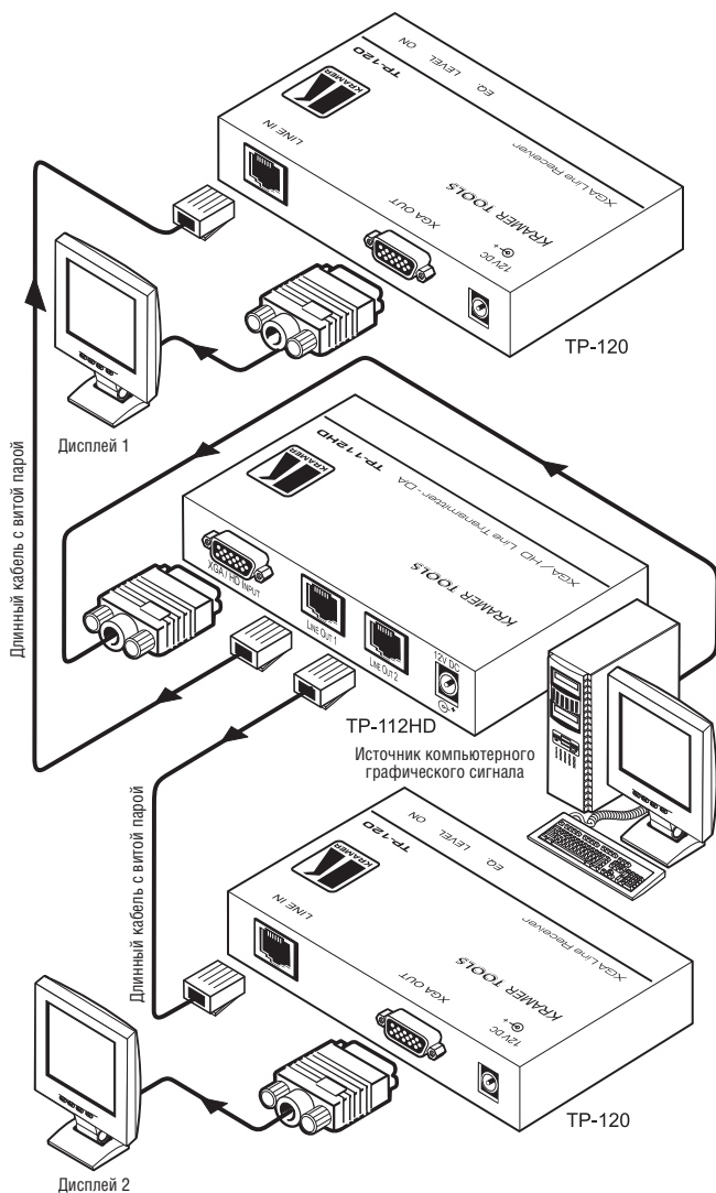
Рис. 5. Распределение сигнала с помощью усилителя-распределителя TP-112HD и двух приемников TP-120
