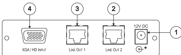
Рис. 3. TP-112HD (нижняя панель)
