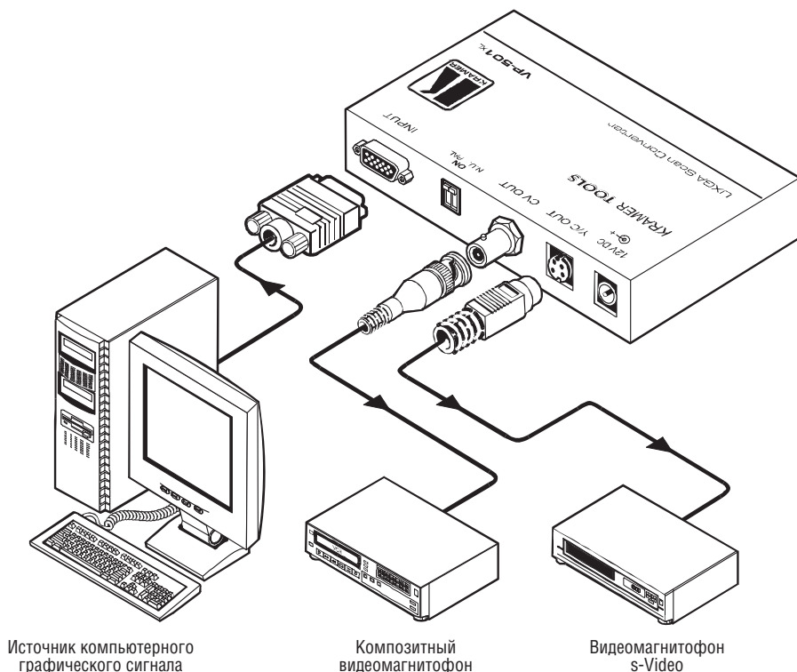
Рис. 3. Подключение VP-501xl
