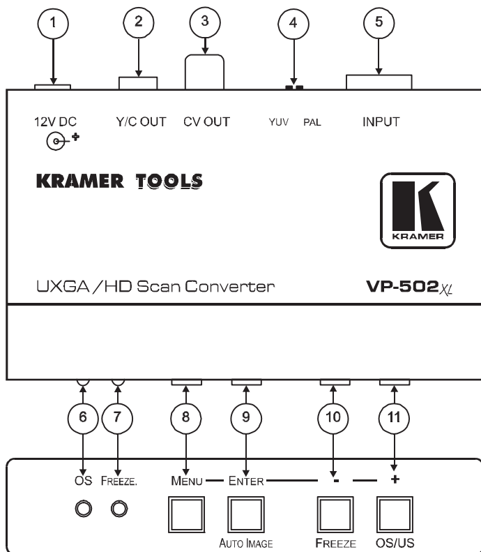
Рис. 2. Преобразователь частоты VP-502xl
